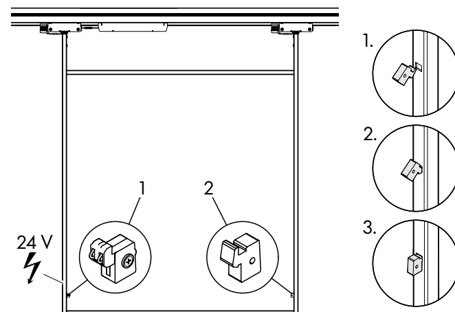
Fig. 81: Support de tablette électrifié (1), non électrifié (2)
