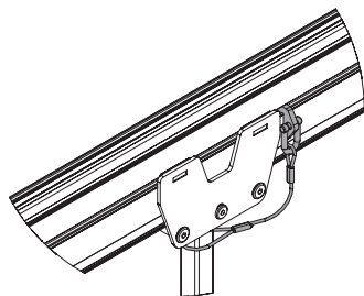
Fig. 43: Installation de l'élément de sécurité
