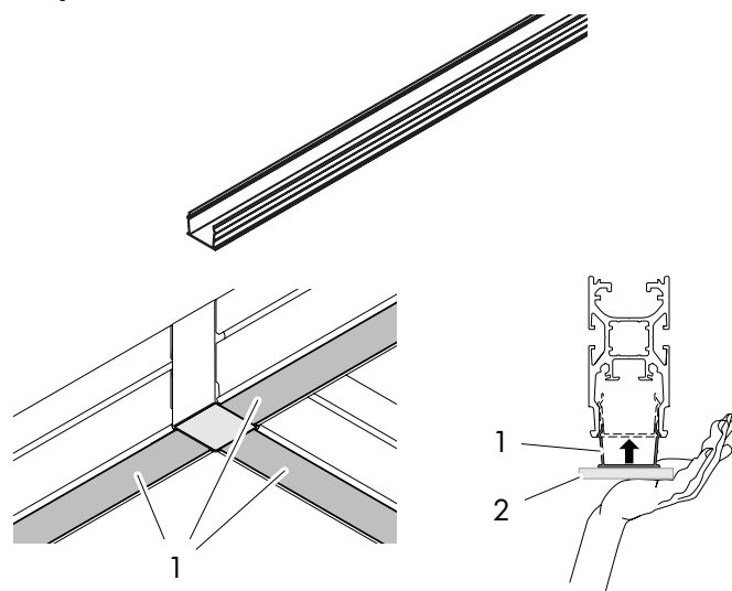
Fig. 21: Montage du profilé de recouvrement (1) avec support souple (2)
