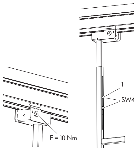
Fig. 55: Serrage
