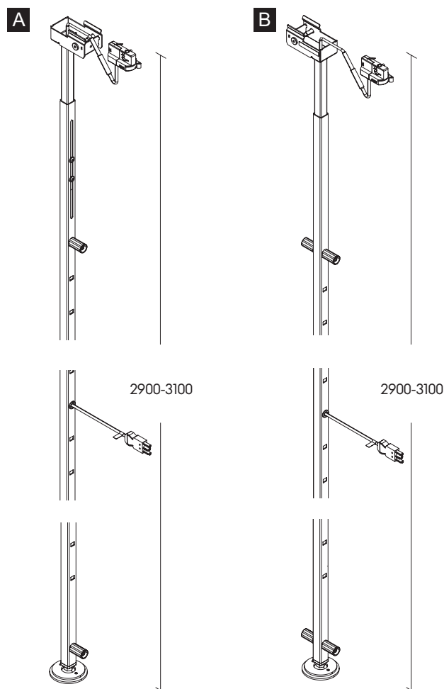
Fig. 59: Assemblage des cadres
