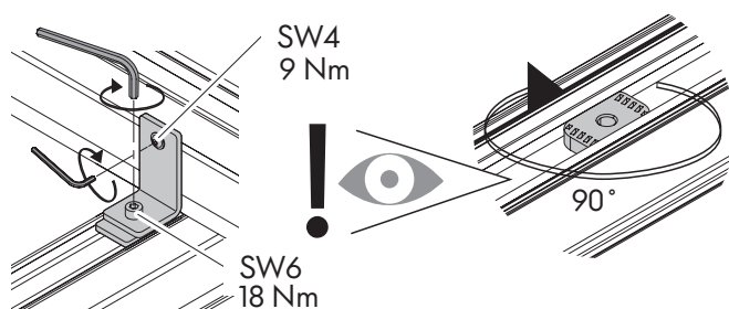
Fig. 18: Montage du kit de fixation
