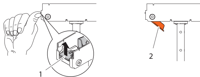
Fig. 26: Préparation de l'adaptateur de suspension
