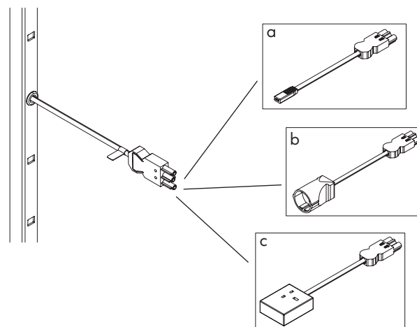
Fig. 61: Tension d'alimentation 120 - 240 V CA
