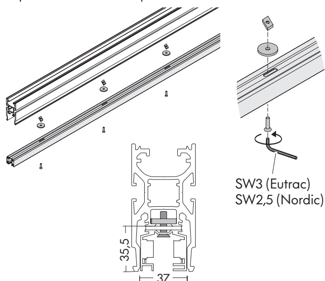
Fig. 24: Mise en place du rail conducteur
