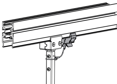
Fig. 35: Bloquer le présentoir et poser un élément de sécurité
