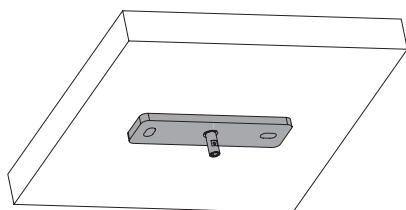
Fig. 6: Vissage de la plaque au plafond
