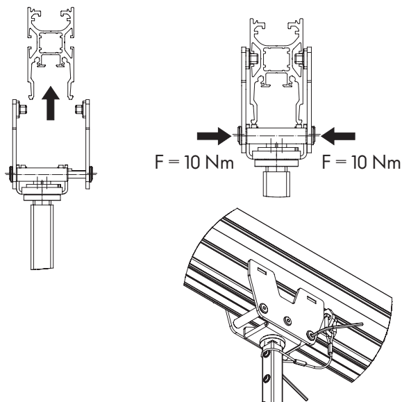
Fig. 42: Fixation du présentoir
